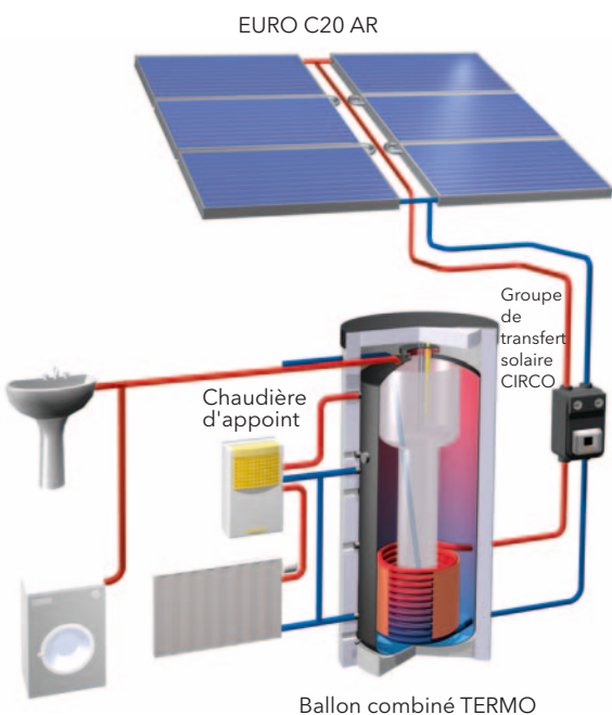
Système solaire combiné COMBligne SH 1440 AD
