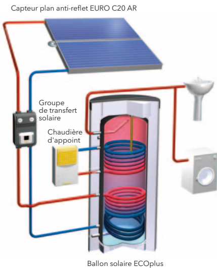
Kit solaire pour eau chaude TOPline BW 480plus AD
